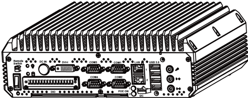
EL1092 (Rx-x0x)
