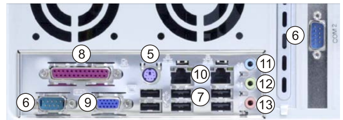
Rückansicht, Beispielkonfiguration
